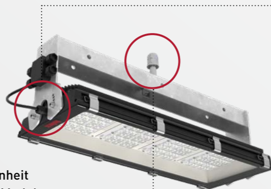
Strahlereinheit mit zwei Modulen 100 000 lm – 120 000 lm
