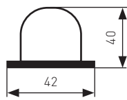
Querschnitt LED-Modul
